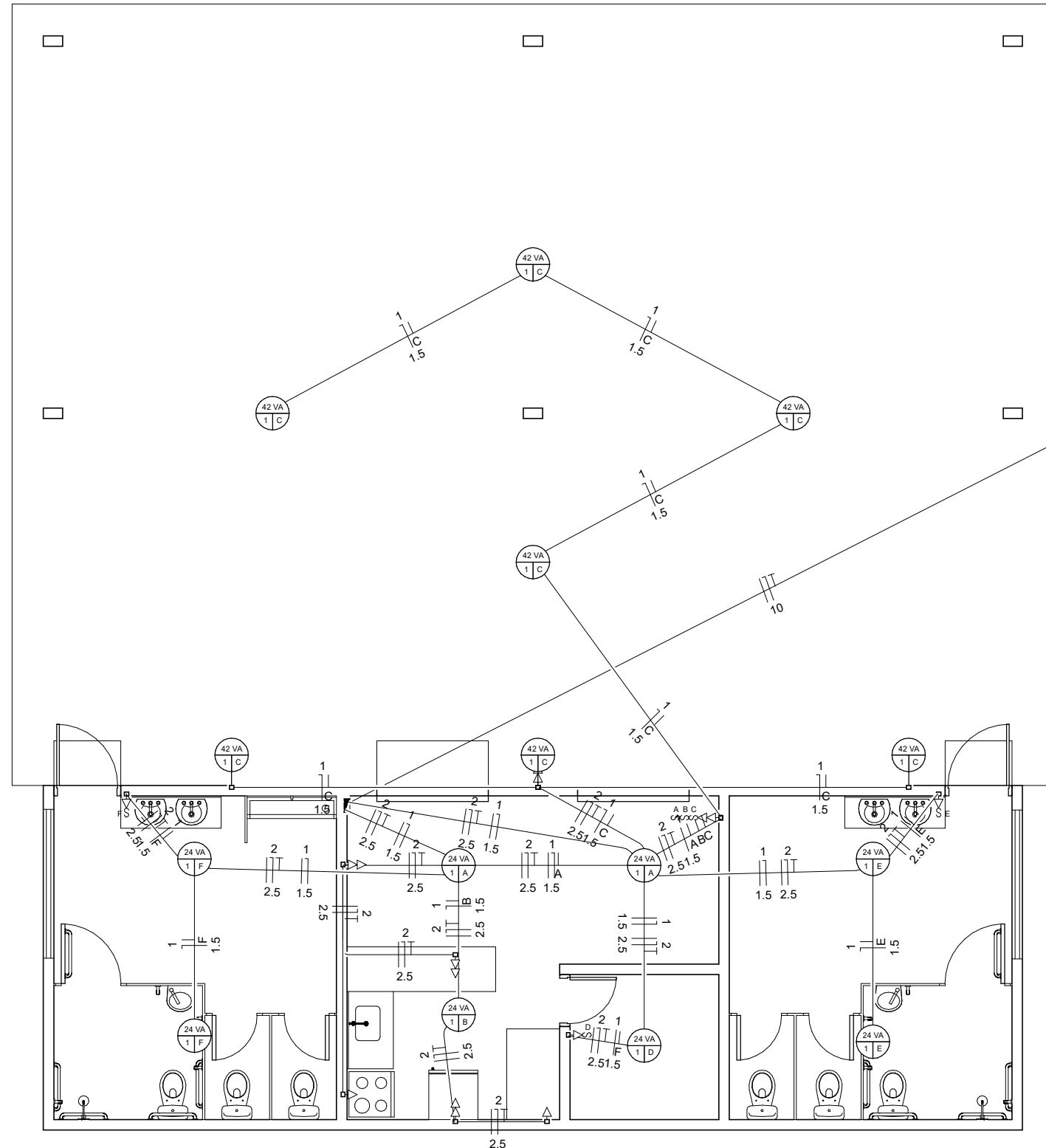
1 PLANTA BAIXA 1 : 75
